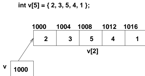
Figura 5.3: Implementación del tipo de dato vector.
