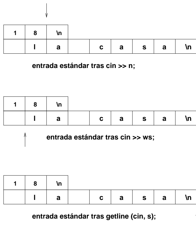
Figura 5.12: Estado de la entrada estándar si se utiliza cin >> ws .
